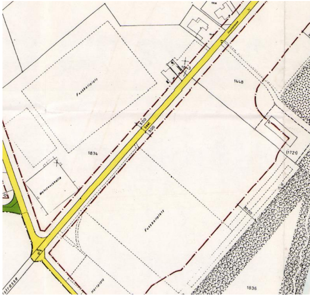
Rechtsgültiger Erschliessungsplan
